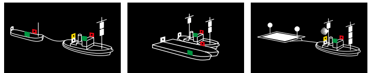
Schleppverbände in Fahrt; Links: bis 200 m Schleplänge (Schlepper nicht über 50 m Länge); Mitte: mit längsseits geschleppten Anhängen; Rechts: über 200 m Länge, mit außergewöhnlichem Schwimmkörper (schleppendes Fahrzeug über 50 m lang)
