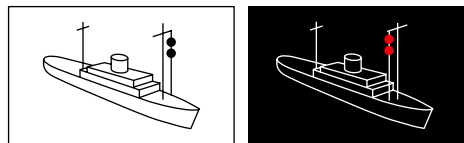
Manövrierfähiges Fahrzeug über 12 m Länge – keine Fahrt durchs Wasser –
