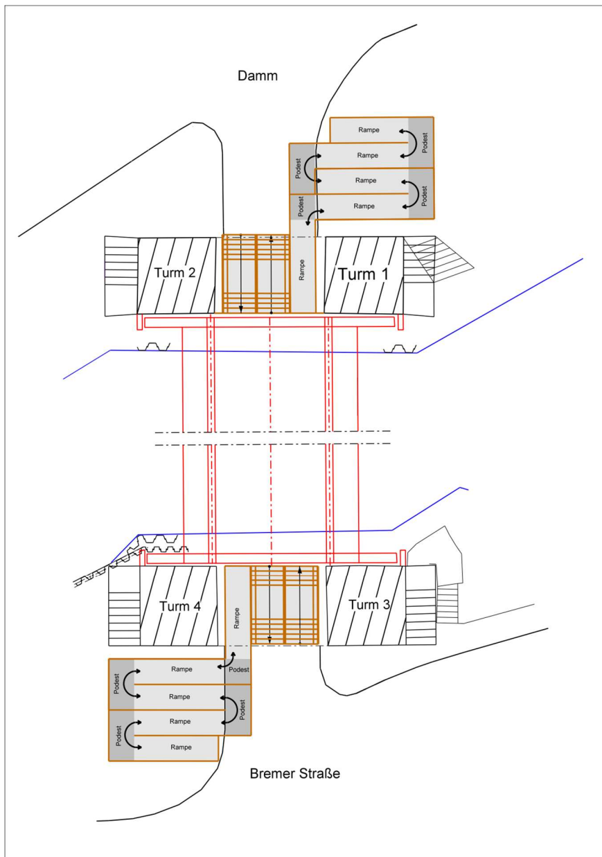
Skizze zu den Treppen und Rampenanlagen
